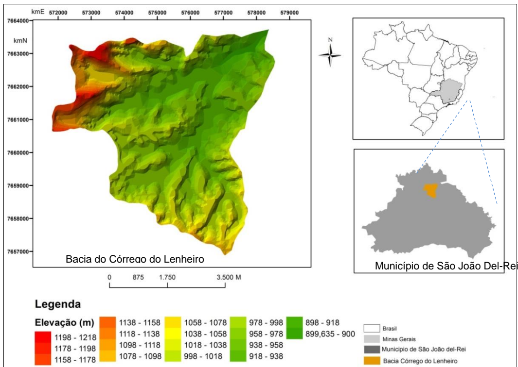
Figura 1: Mapa hipsométrico da bacia do Córrego do Lenheiro e sua localização em São João Del-Rei - MG
